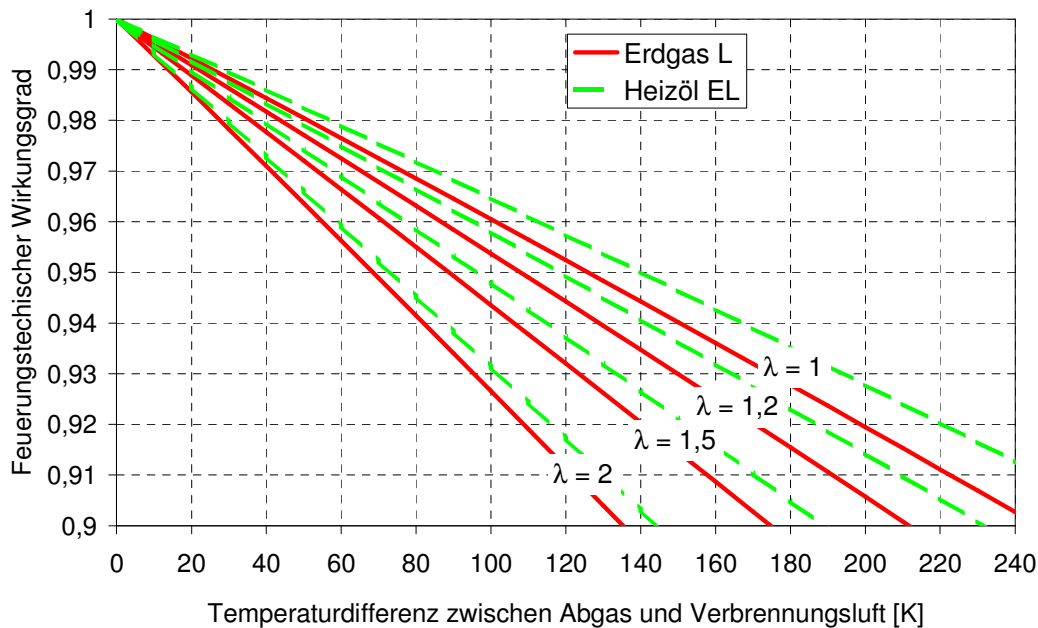
Bild 3-10: Feuerungstechnischer Wirkungsgrad
