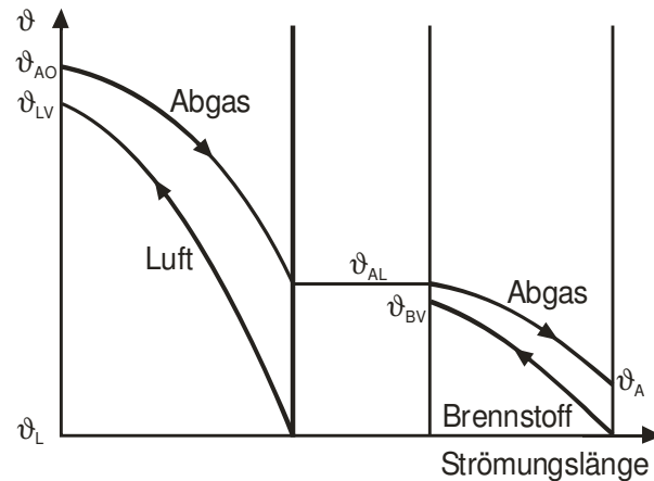
Bild 3-14: Prinzip der Luft- und Brennvorwärmung
