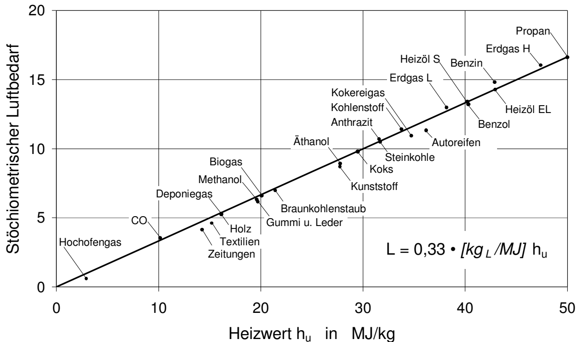
Bild 3-2: Zusammenhang zwischen Heizwert und Luftbedarf in kg L/kg B
