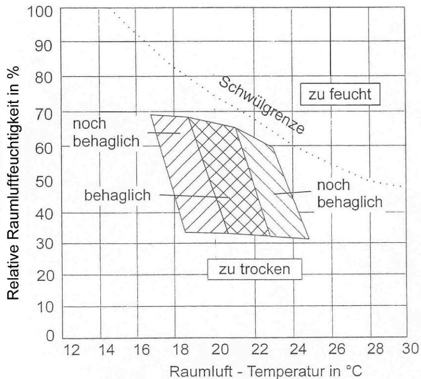
Bild 4: Behaglichkeitsfeld Raumlufttemperatur/rel. Luftfeuchtigkeit
